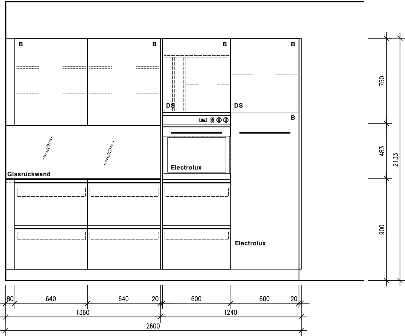
Ansicht A
