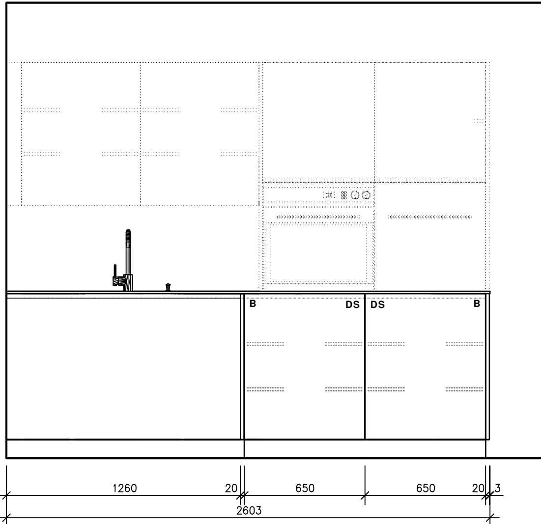
Ansicht C
