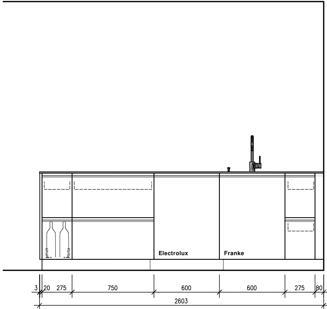
Ansicht B
